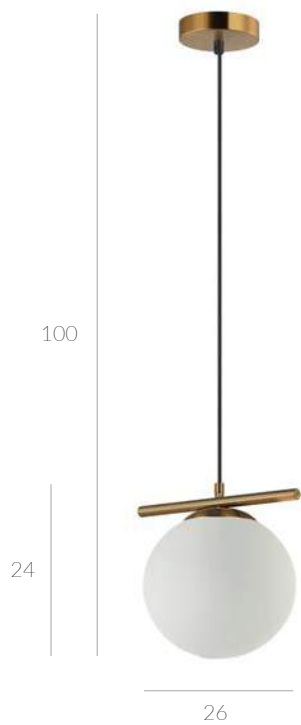
PND-463321L-BRO+W Ø E14 1x40W
