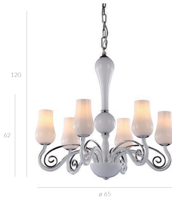
MD10904-6A Ø E14 6x40W
