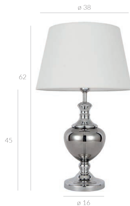
TB-6620-1 ♀ E27 1x60W
