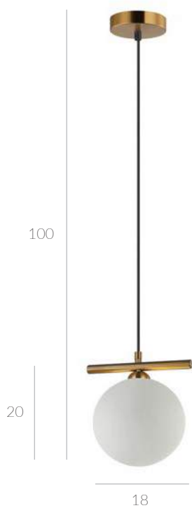
PND-463321M-BRO+W Ø G9 1x25W
