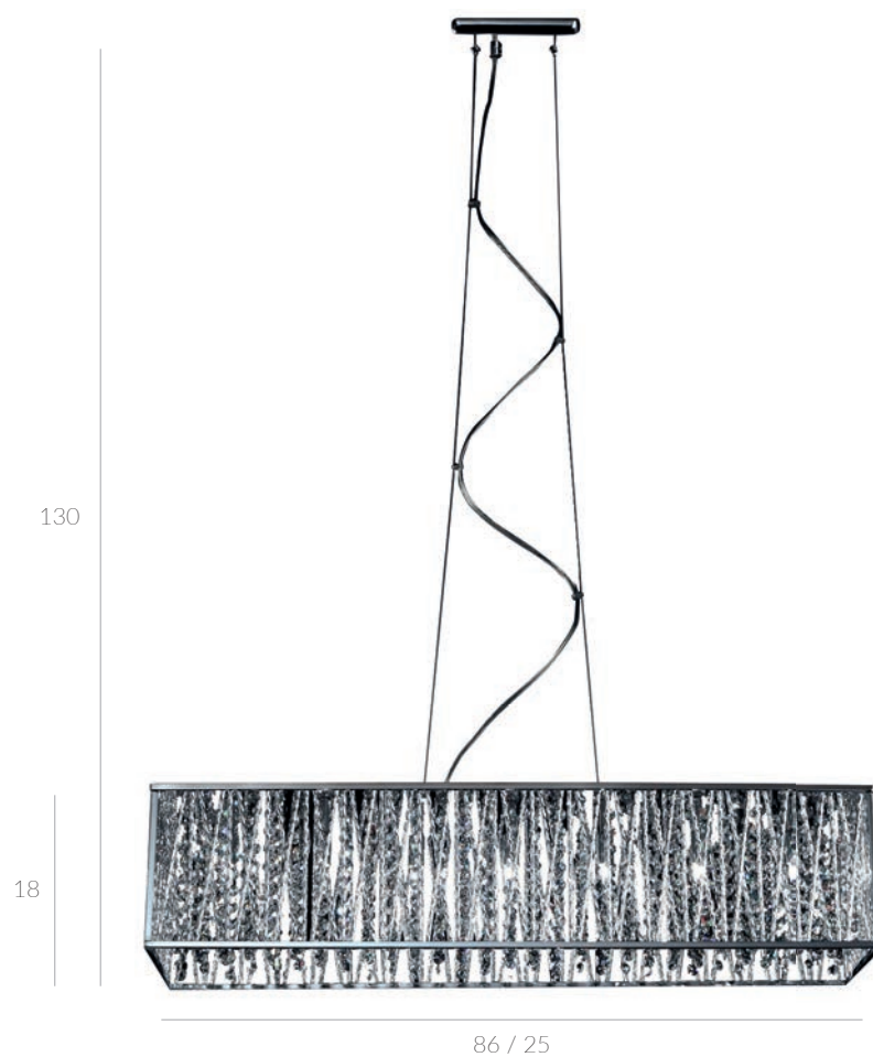
P0282-07L-F4QL ⌀ G9 7x42W
